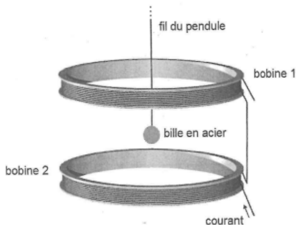
Bobines de Helmholtz
