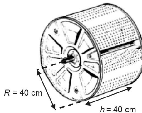
Figure 2. Schéma du tambour du lave-linge
